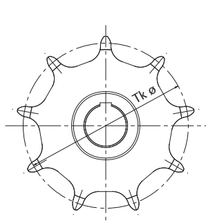
Abbildung 42: HEKO Kettenrad Typ VIE-B einteiliges, innenverzahntes, geschweißtes Kettenrad mit mechanisch bearbeiteter Kettenauflage Nabe aus Stahl, Zahnkranz aus legiertem CrMo-Stahl
