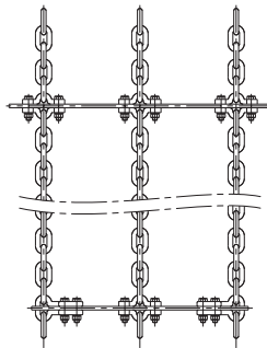
Abbildung 16: Dreistrangkette mit Befestigungshälften
