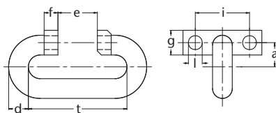
Abbildung 21: HEKO Befestigungsglieder Typ BGQ
