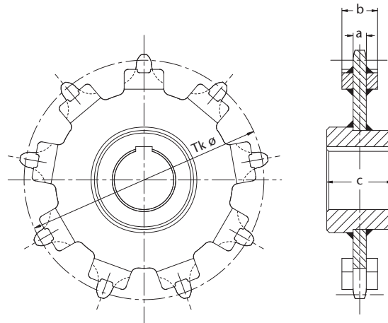
Abbildung 45: HEKO Kettenrad Typ GIE, innenverzahntes, einteiliges Kettenrad mit angeschweißter Kettenauflage
