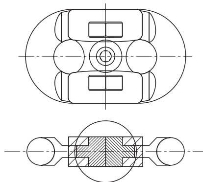
Abbildung 35: Kettenschloss Typ HR
