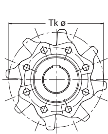
Abbildung 58: HEKO Kettenrad Typ RLA für Gabellaschenkettentyp Modell 69226
