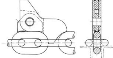
Abbildung 33: Mitnehmer mit Ausklinkvorrichtung für Reversierbetrieb
