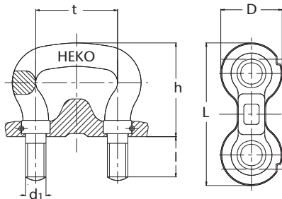
Abbildung 61: HEKO Kettenbügel Typ TS
