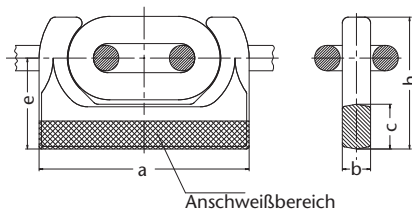
Abbildung 19: HEKO Steckmitnehmer SMO
