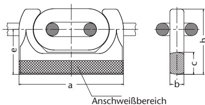
Abbildung 63: HEKO Steckmitnehmer Typ SMO
