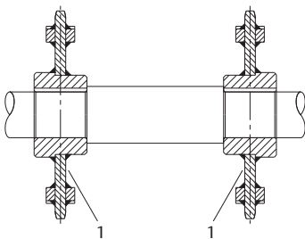
Abbildung 68: Montagehinweis 1
