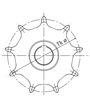
Abbildung 41: HEKO Kettenrad Typ VIE-A innenverzahntes, einteiliges Kettenrad mit mechanisch bearbeiteter Kettenauflage komplett aus legiertem CrMo-Stahl
