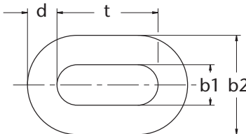
Abbildung 61: HEKO Kettenbügel Typ TS
