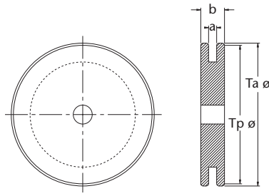
Abbildung 59: HEKO Kettenrad Typ RLE unverzahnt für Laschenkettentyp
