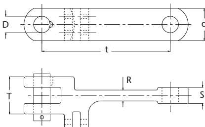
Abbildung 56: HEKO Gabellaschenketten, gesenkgeschmiedet, Doppelstrang
