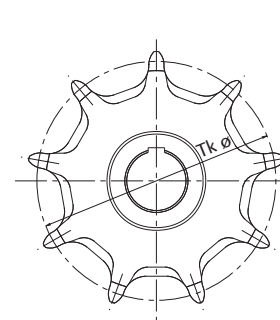
Abbildung 43: HEKO Kettenrad Typ VIE-C und VIE-D mit angeschrägten Ausfallöffnungen – aus dem Vollen gedreht bzw. in geschweißter Ausführung (alternativ zu VIE-A und VIE-B)
