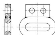
Abbildung 27: angeschweißte Mitnehmer zur Aufnahme verschiedener Vorrichtungen
