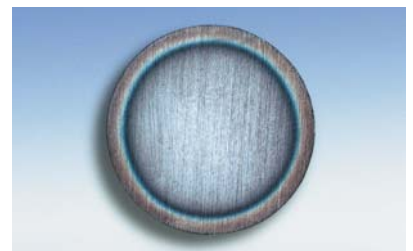
Abbildung 4 : Querschnitt durch ein einsatzgehärtetes Kettenglied.
