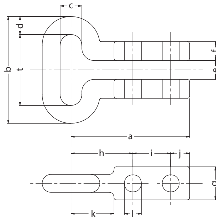
Abbildung 10: HEKO Spezialglied Typ SP
