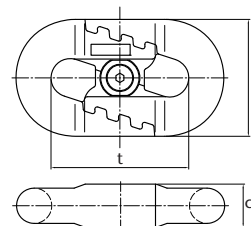
Abbildung 64: Kettenschloss Typ HF
