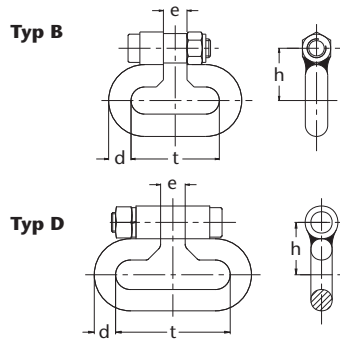
Abbildung 36: Kettenschloss Typ B mit angeschweißter Mutter, Typ D mit loser Mutter
