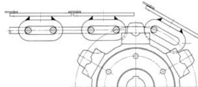
Abbildung 32: Plattenbandförderer als Förderband, geschlossen
