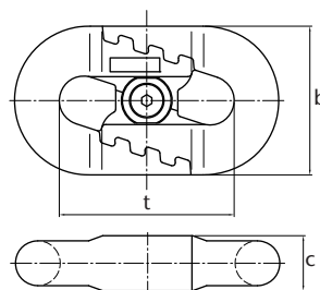
Abbildung 39: Kettenschloss Typ HF
