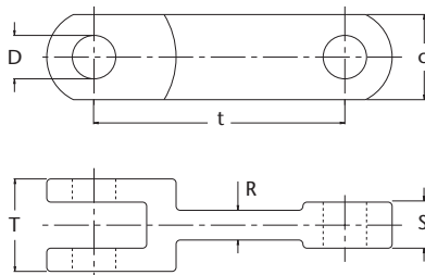
Abbildung 55: HEKO Gabellaschenketten, gesenkgeschmiedet, Einzelstrang
