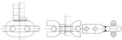
Abbildung 25: angeschweißte Mitnehmer für innenverzahnte und taschenverzahnte Kettenräder in Zweistranganlagen zum Anschrauben der Mitnehmer Typ AFS
