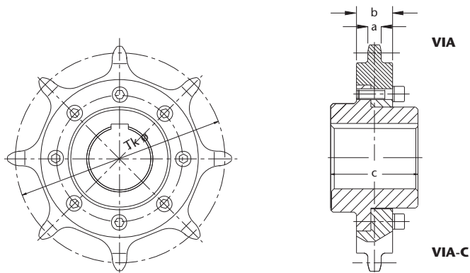
Abbildung 40: Innenverzahntes austauschbares HEKO Kettenrad Typ VIA bzw. VIA-C mit angeschrägten Ausfallöffnungen
