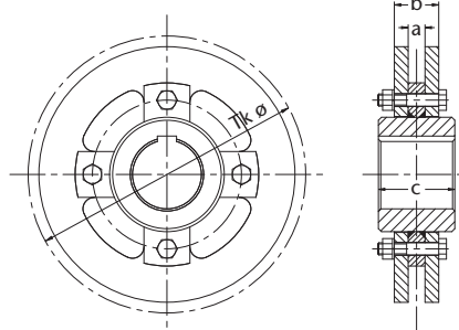
Abbildung 53: HEKO Kettenrad unverzahnt in Stahlausführung Typ GUA – austauschbar
